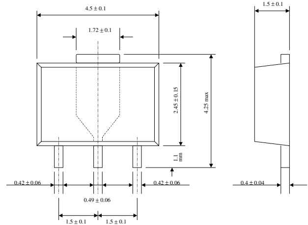
SOT-89 :
